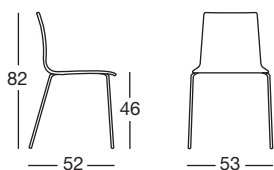
Struttura a 4 gambe 4-leg frame Art. 2675
